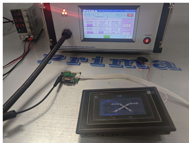
图 5-2 ESD 测试图
