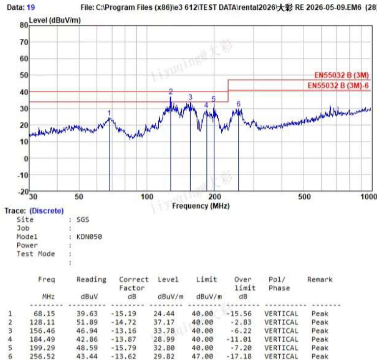
图 5-7 RE 测试垂直方向
