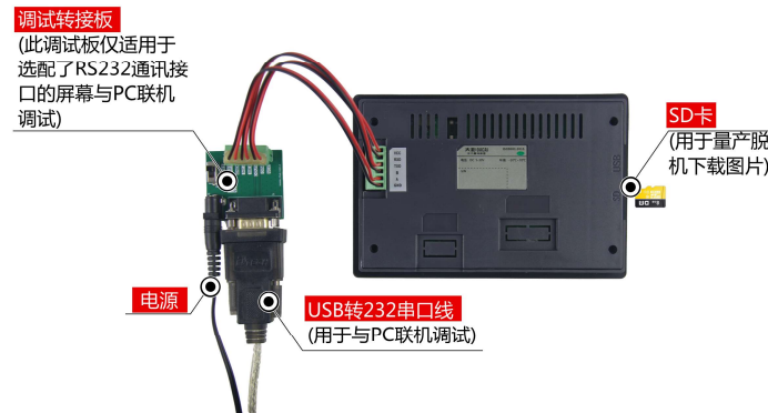
图 1-5 RS232 调试工具图
