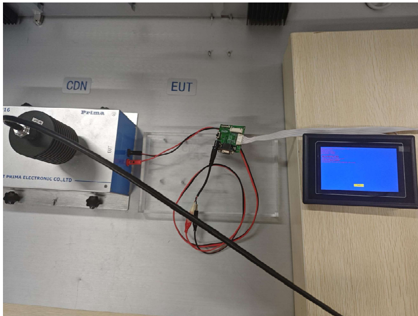
图 5-4 CS 测试图
