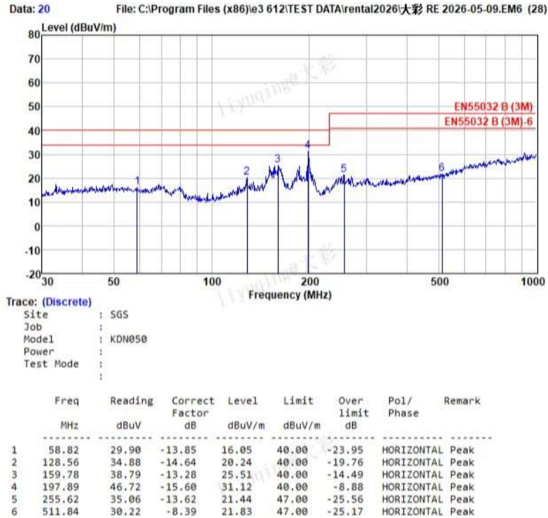
图 5-6 RE 测试水平方向
