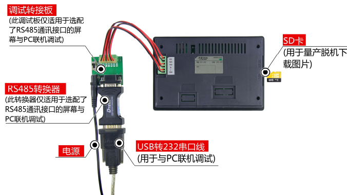
图 1-6 RS485 调试工具图
