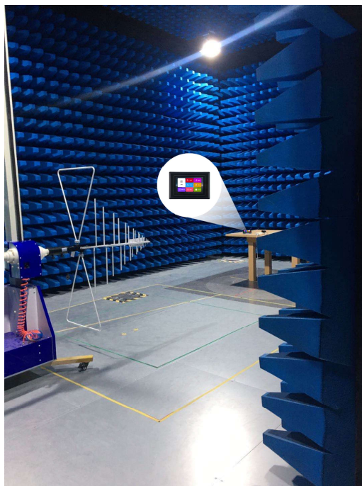
图 5-5 RE 测试图
